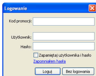
Okno logowania
